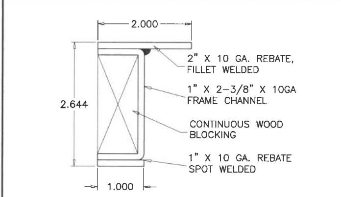
2 PIVOT JAMB ASSEMBLY
