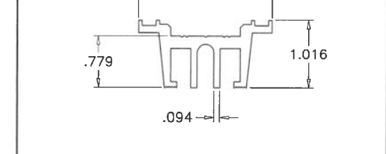
6063-T5 EURO-24 PIVOT ADAPTER
