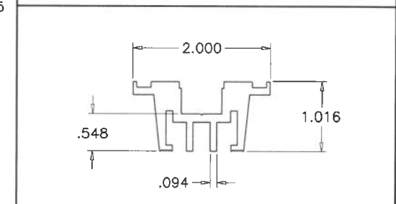
6063-T5 EURO-25 LOCK JAMB ADAPTER
